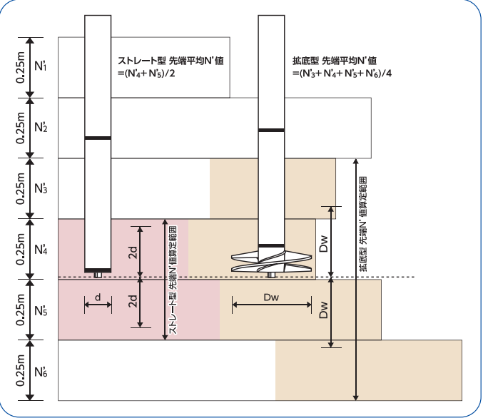
図1. 先端平均N'値の算定範囲
